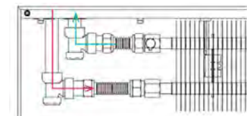
Uzun kenardan bağlantı
